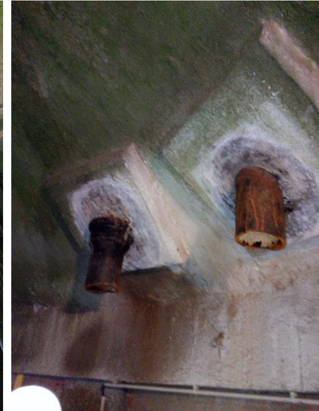
Découpage des tuyauteries dans la cuve et au niveau supérieur du château d'eau
